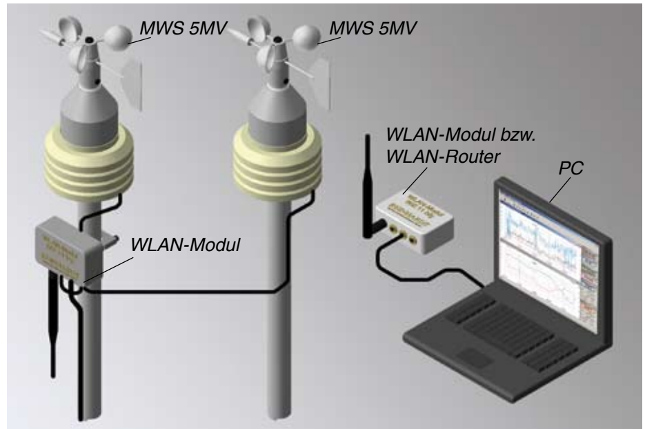
Datenübertragung mit WLAN-Netz
